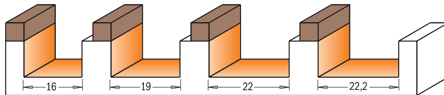
Tegning er 1:1
